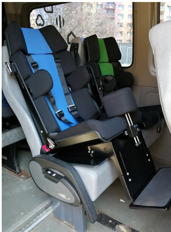
Umístění speciálních sedaček pro klienty na sedadlech.
