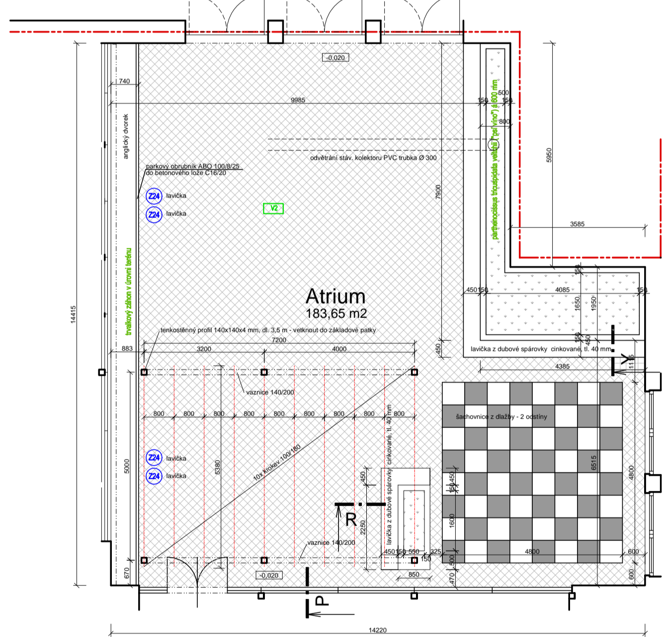
Půdorys atria
