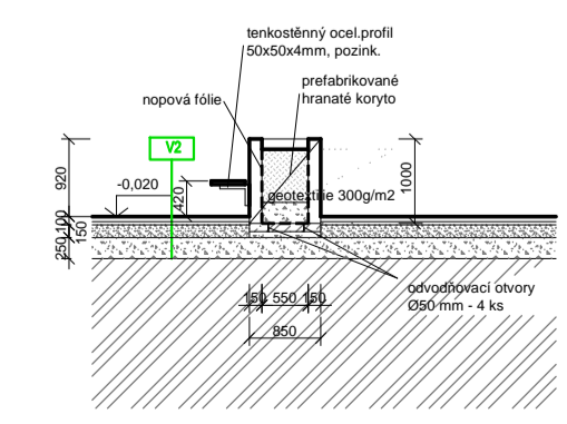
Řez květinovým korytem R-R
