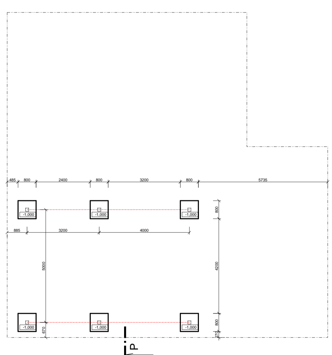
Půdorys základů pergoly v atriu
