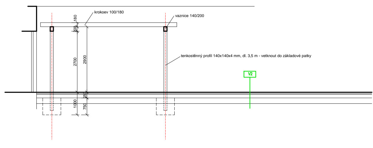
Řez pergolou P-P
