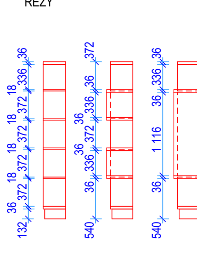
ŘEZY
