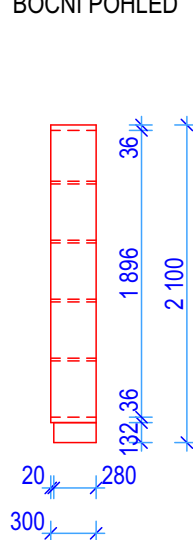
BOČNÍ POHLED
